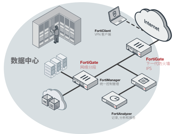
FortiGate 7000E 系列在数据中心的部署 (IPS / NGFW, 基于意图的网络分段)
